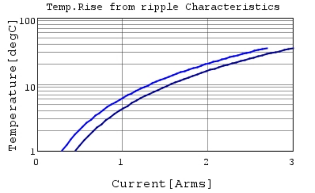
GRM185R61E105KA12 Temp.rise — 500kHz —
