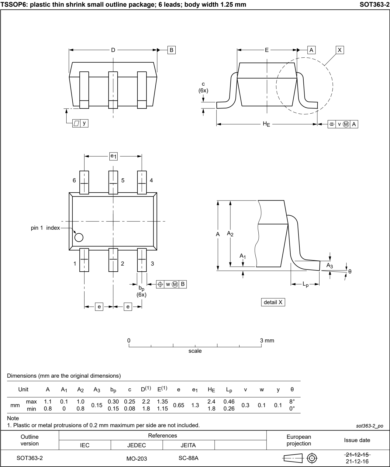
Fig. 10. Package outline SOT363-2 (TSSOP6)
